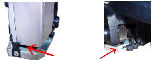
帯鉄幅変更用ガイド 16mmと19mm幅の切替が出来ます
